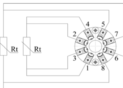
Рисунок 6в - ТС с двумя элементами и четырехпроводной схемой рассоединения (2x4)
