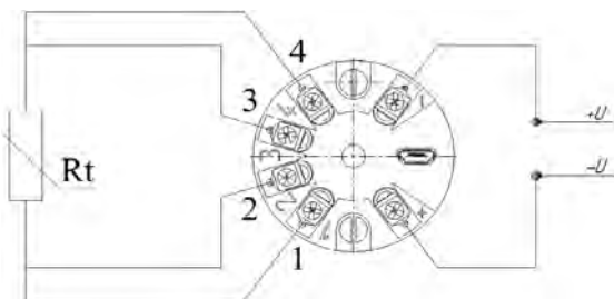
Рисунок 7в - ТС-Б-У с четырехпроводной схемой рассоединения (x4)
