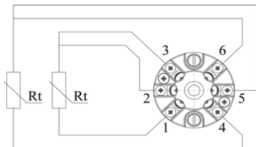
Рисунок 5в - ТС с двумя элементами и трехпроводной схемой рассоединения (2x3)
