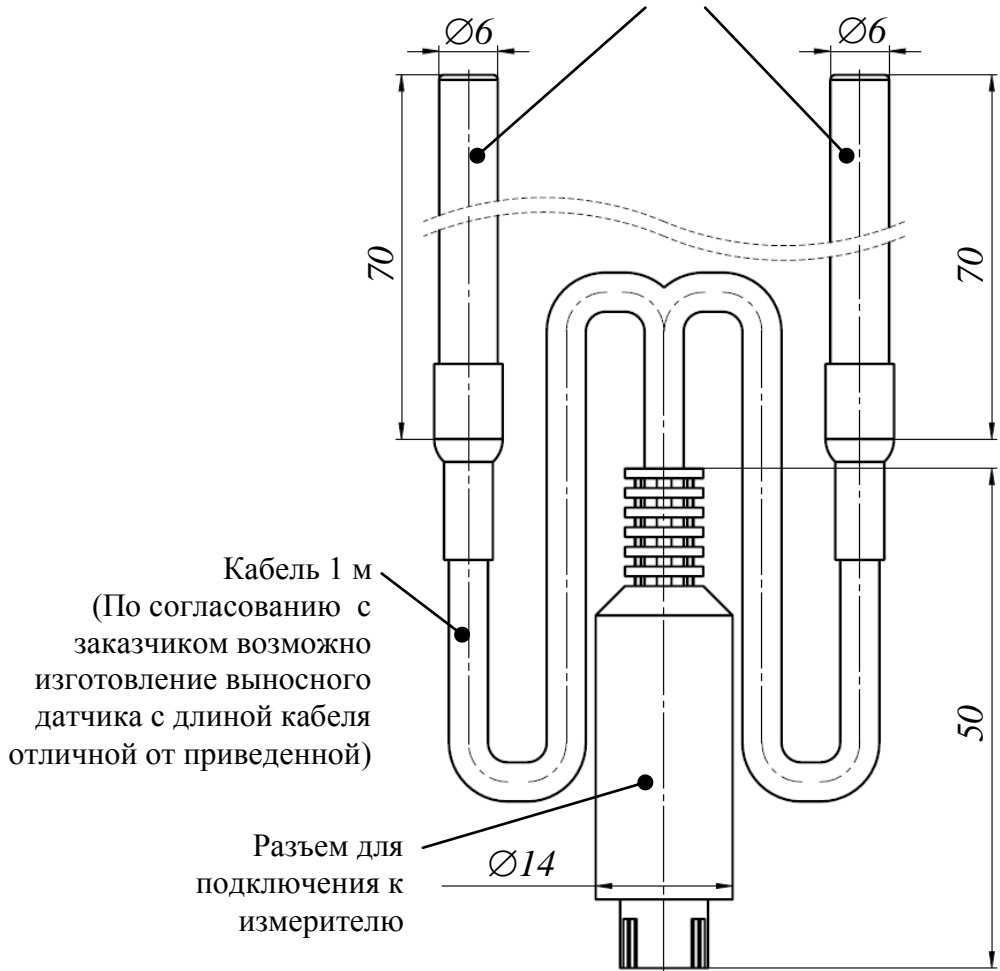
Внешний вид выносных датчиков температуры
